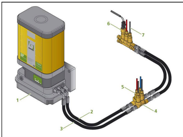
Twin system med pump, matarledning och fördelningsblock
