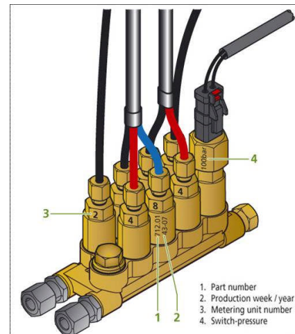
Doseringsblock med ventiler och tryckvakt
